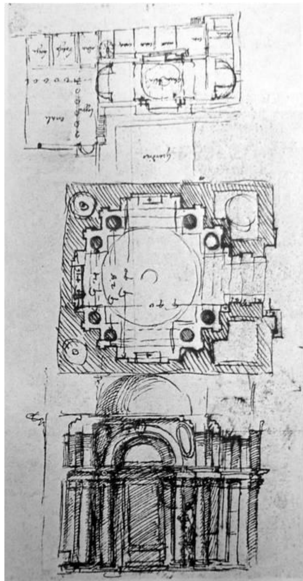
Girolamo Rainaldi, disegno di progetto per la basilica di Loreto, particolare di due cappelle (ASPr, Raccolta Mappe e disegni, Vol. 49, f. 39),
